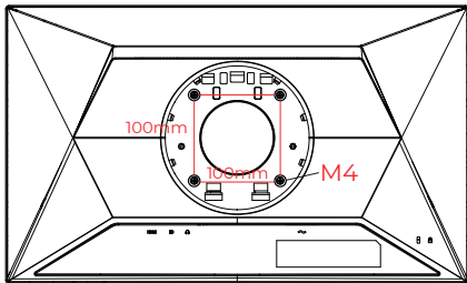
벽걸이 나사 사양: M4*(10+X)mm (X=벽걸이 브래킷 두께)
