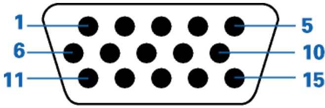
15핀 컬러 디스플레이 신호 케이블
